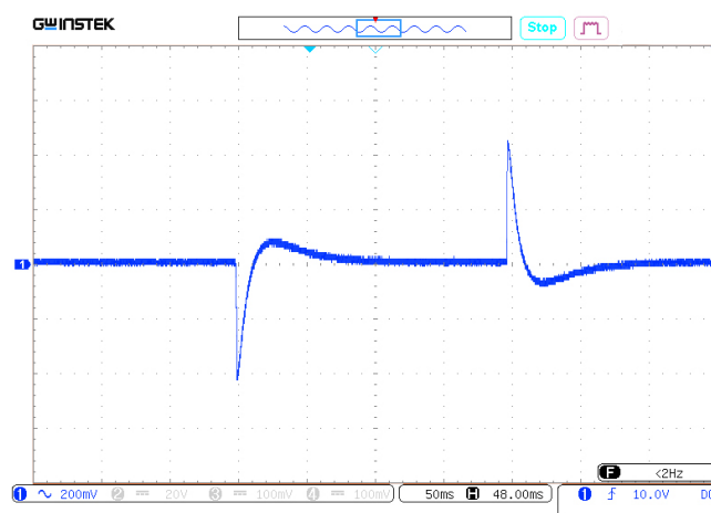
Рис. 28. Осциллограмма переходного отклонения выходного напряжения при изменении выходного тока с 50% до 100 %. Масштаб 200 мВ/дел. Развертка 50 мс/дел.
