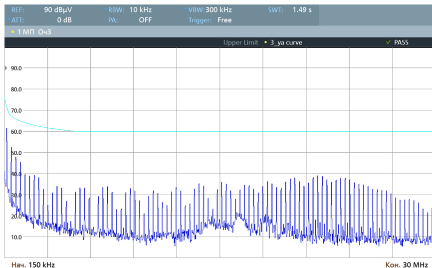
Рис. 33. Диапазон 0,15..30 МГц.
