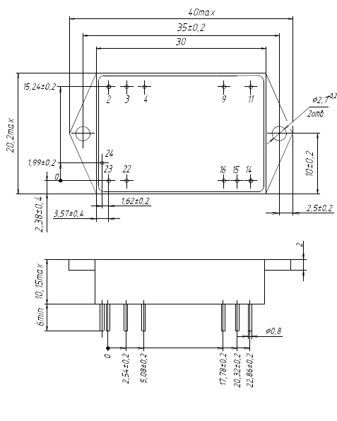
Рис. 34. Модуль одноканальный в корпусе с фланцами (индекс «У»).
