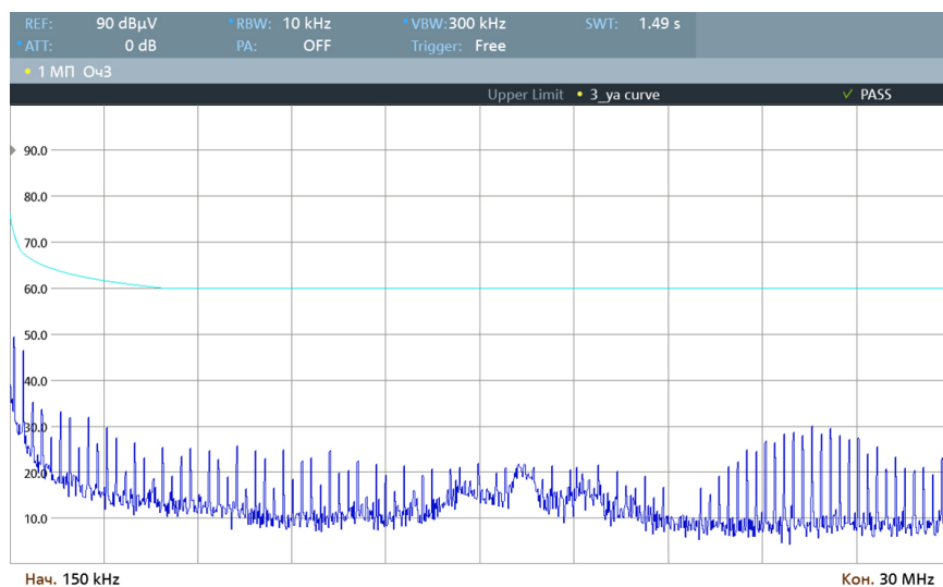
Рис. 32. Диапазон 0,15..30 МГц.
