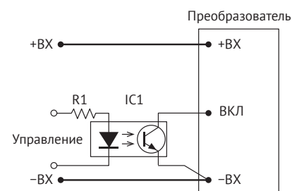
Рис. 8. ВКЛ/ВЫКЛ с помощью оптрона.
