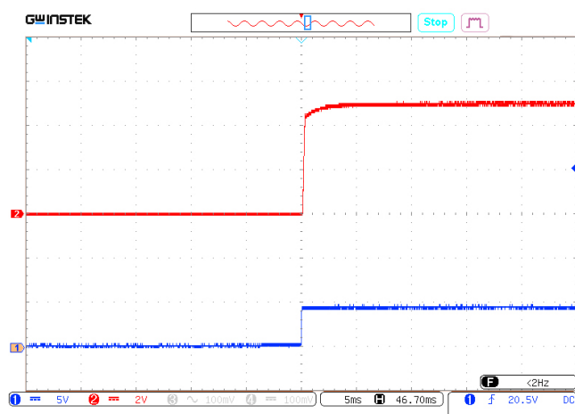
Рис. 21. Осциллограмма установления выходного напряжения с момента подачи команды дистанционного управления. Луч 1 (синий) — напряжение на выходе «ВКЛ». Масштаб 5 В/дел. Луч 2 (красный) — выходное напряжение. Масштаб 2 В/дел. Развертка 5 мс/дел.
