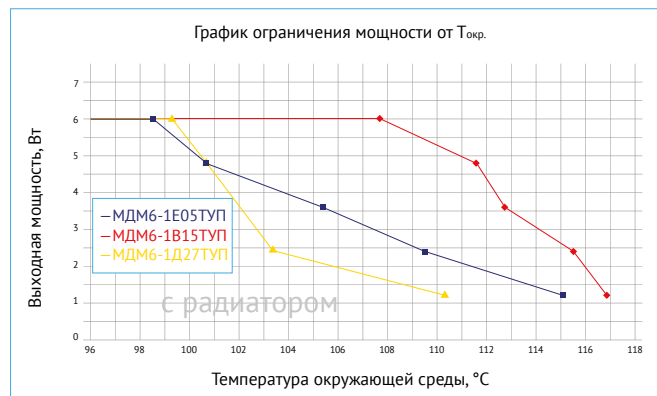
Рис. 20. График ограничения мощности от T_{ОКР.} с применением радиатора БКЯЮ.752694.008 ( S=74 \text{ см}^2 ).
