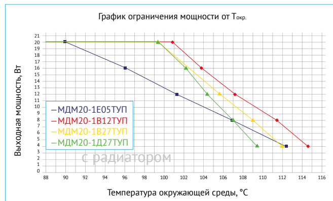
Рис. 19. График ограничения мощности от T_{ОКР.} с применением радиатора БКЯЮ.752695.054 ( S=94 \text{ см}^2 ).
