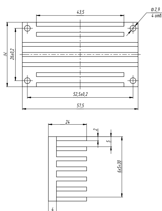
Рис. 45. БКАЮ.752695.262-01.
