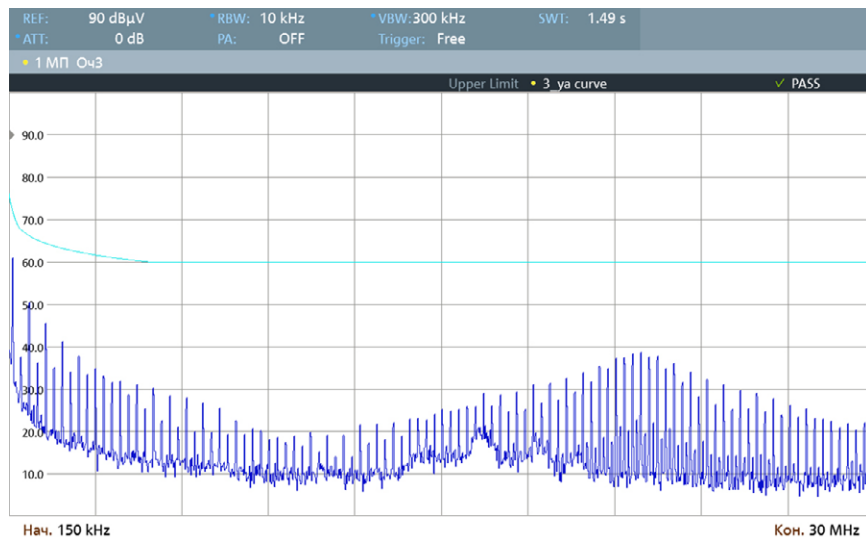
Рис. 31. Диапазон 0,15..30 МГц.
