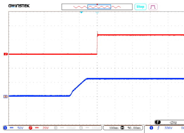
Рис. 25. Осциллограмма установления выходного напряжения с момента подачи входного напряжения. Луч 1 (синий) — входное напряжение. Масштаб 50 В/дел. Луч 2 (красный) — выходное напряжение. Масштаб 20 В/дел. Развертка 100 мс/дел.
