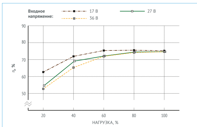
Рис. 11. МДМ20-1B05ТУП.
