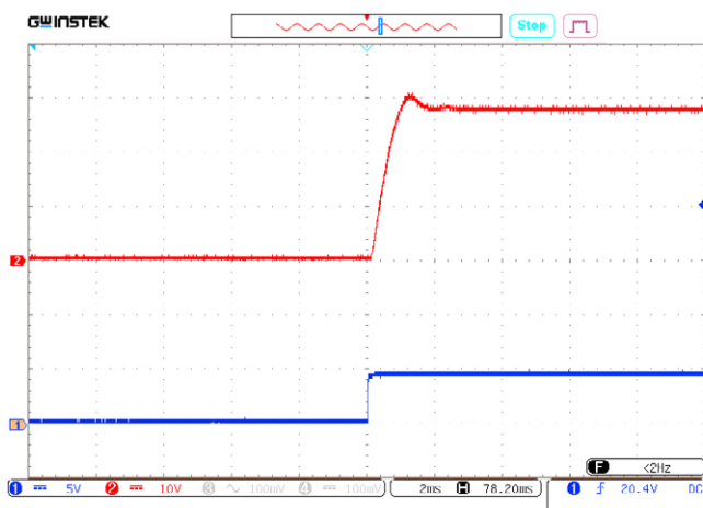
Рис. 24. Осциллограмма установления выходного напряжения с момента подачи команды дистанционного управления. Луч 1 (синий) — напряжение на выводе «ВКЛ». Масштаб 5 В/дел. Луч 2 (красный) — выходное напряжение. Масштаб 10 В/дел. Развертка 2 мс/дел.
