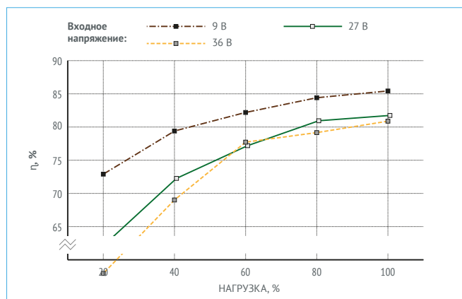
Рис. 17. МДМ25-1Е27ТУП.
