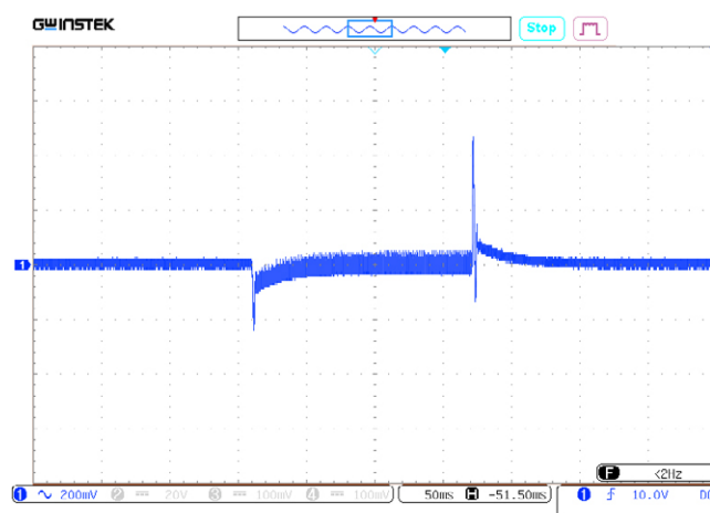
Рис. 30. Осциллограмма переходного отклонения выходного напряжения при изменении выходного тока с 50% до 100%. Масштаб 200 мВ/дел. Развертка 50 мс/дел.
