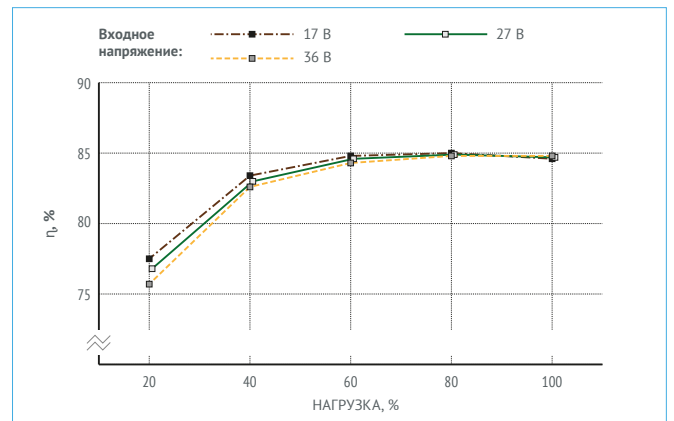
Рис. 14. МДМ120-1В12ТУП.
