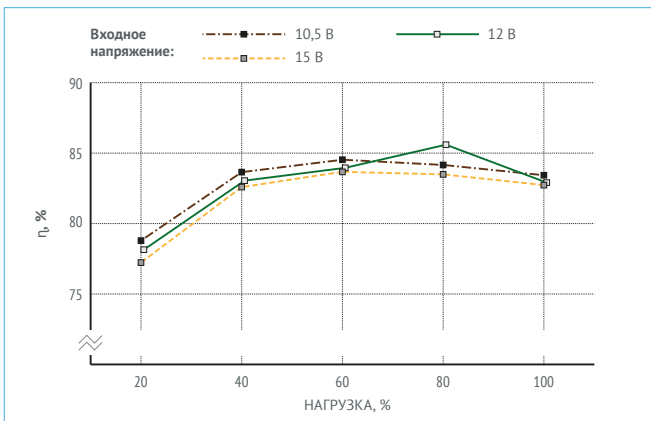
Рис. 13. МДМ120-1А15ТУП.
