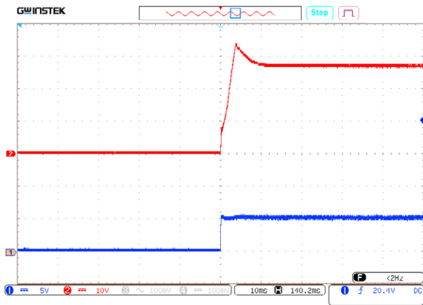
Рис. 24. Осциллограмма установления выходного напряжения с момента подачи команды дистанционного управления. Луч 1 (синий) – напряжение на выводе «VKЛ». Масштаб 5 В/дел. Луч 2 (красный) – выходное напряжение. Масштаб 10 В/дел. Развертка 10 мс/дел.
