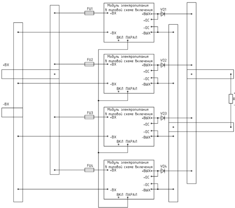
Рис. 10. Схема подключения модулей электропитания для параллельной работы (без указания элементов типовой схемы подключения [Рис. 2]).
