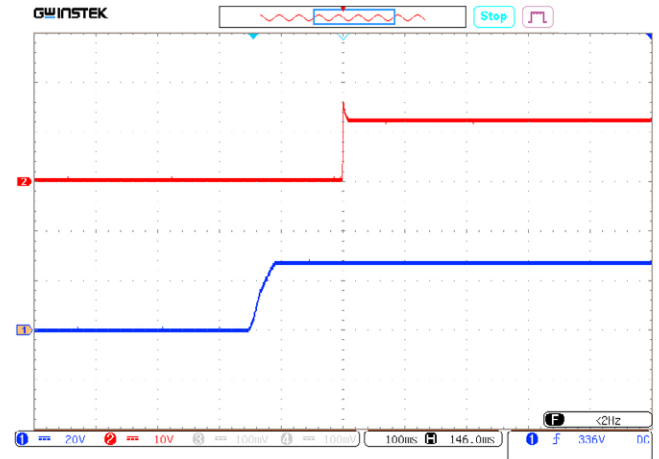
Рис. 22. Осциллограмма установления выходного напряжения с момента подачи входного напряжения. Луч 1 (синий) – входное напряжение. Масштаб 20 В/дел. Луч 2 (красный) – выходное напряжение. Масштаб 10 В/дел. Развертка 100 мс/дел.
