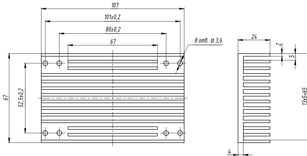
Рис. 31. БКЯЮ.752695.265-01.
