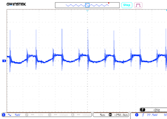
Рис. 23. Осциллограмма пульсаций выходного напряжения. Масштаб 5 мВ/дел. Развертка 5 мкс/дел.
