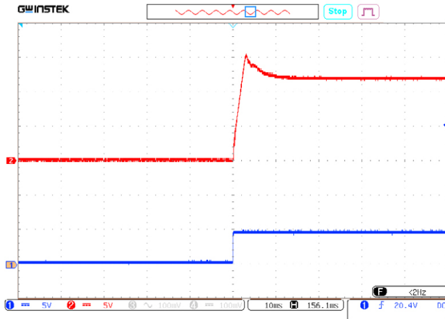
Рис. 21. Осциллограмма установления выходного напряжения с момента подачи команды дистанционного управления. Луч 1 (синий) – напряжение на выводе «ВКЛ». Масштаб 5 В/дел. Луч 2 (красный) – выходное напряжение. Масштаб 5 В/дел. Развертка 10 мс/дел.
