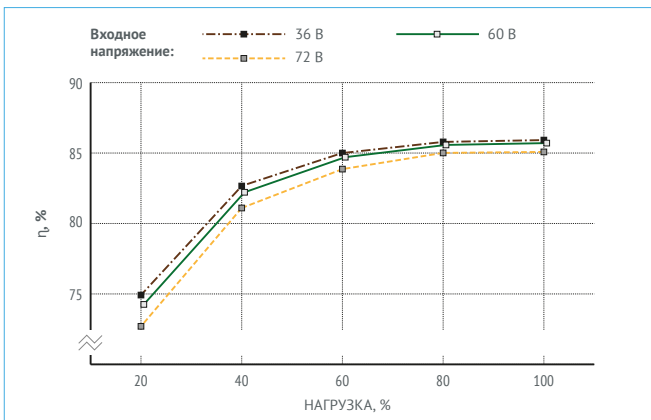
Рис. 17. МДМ160-1Д15ТУП.
