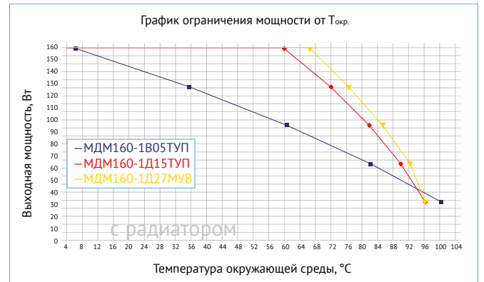
Рис. 20. График ограничения мощности от T_{окр.} с применением радиатора БКЯЮ.752695.265-01 ( S=631 \text{ см}^2 ).
