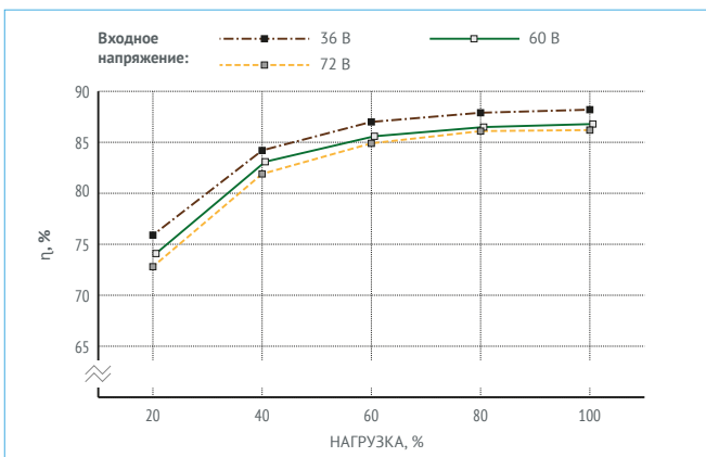
Рис. 18. МДМ160-1Д27ТУП.
