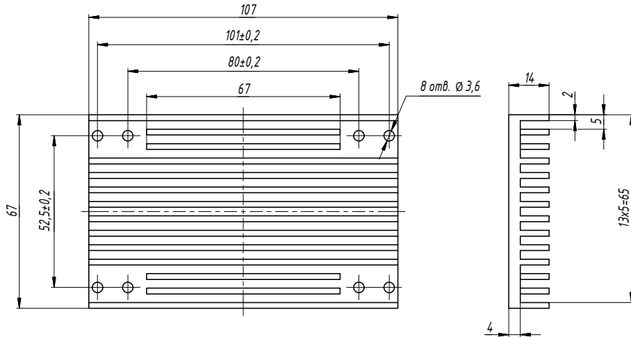
Рис. 30. БКЯЮ.752695.265.
