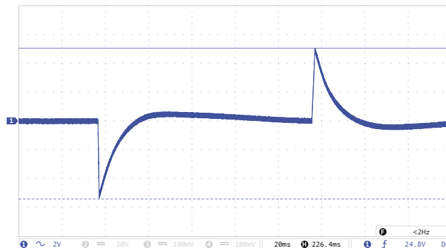
Рис. 20. Осциллограмма переходного отклонения выходного напряжения при изменении выходного тока с 50% до 100%.
