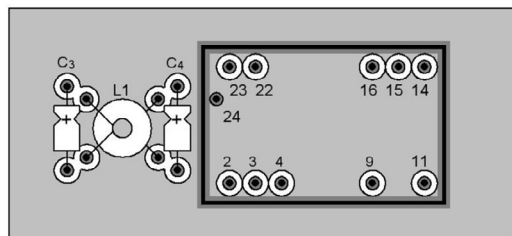
Рис. 3. Вид сверху.
