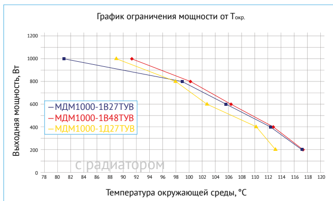
Рис. 16. График ограничения мощности от T_{окр} с применением радиатора БКЯЮ.752695.067 ( S=1890\text{ см}^2 ) с принудительным обдувом, скорость воздушного потока 3,5 м/с. Для разных исполнений модулей.
