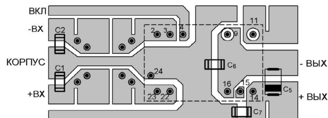
Рис. 4. Вид снизу.
