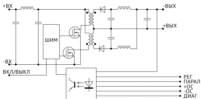
Рис. 1. Функциональная схема МДМ1000-П.
