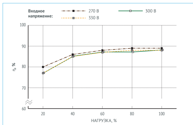
Рис. 20. МДМ340-1Ф09ТУА.
