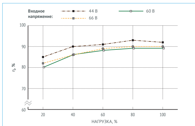
Рис. 17. МДМ340-1Э36ТУА.
