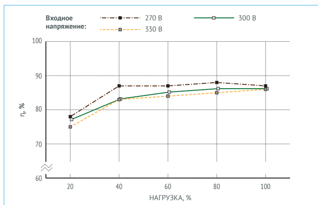
Рис. 19. МДМ340-1Ф7,5ТУА.
