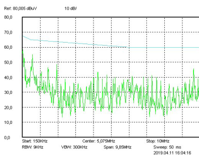
Рис. 71. Диапазон 0,15–10 MHz.
