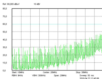
Рис. 63. Диапазон 10–30 МГц.
