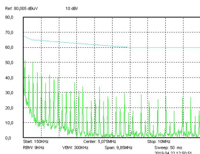
Рис. 68. Диапазон 0,15–10 МГц.
