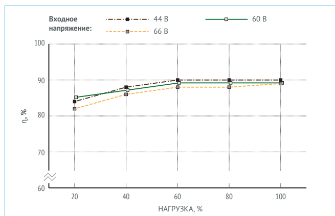
Рис. 16. МДМ340-1Э28ТУА.
