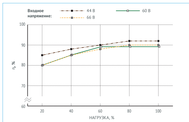
Рис. 18. МДМ340-1Э50ТУА.
