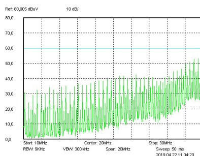
Рис. 66. Диапазон 10–30 МГц.
