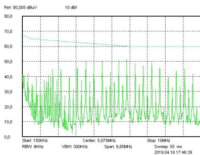
Рис. 74. Диапазон 0,15–10 MHz.
