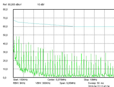
Рис. 62. Диапазон 0,15–10 МГц.
