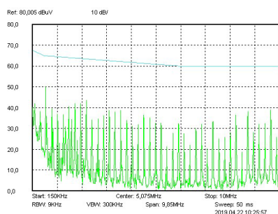
Рис. 65. Диапазон 0,15–10 МГц.
