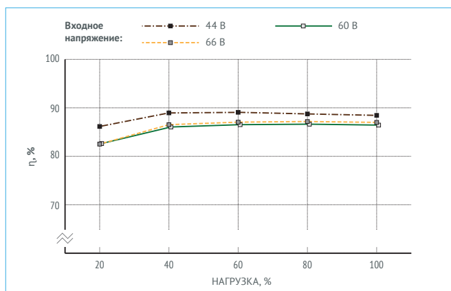
Рис. 15. МДМ340-1Э12ТУА.
