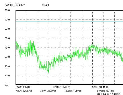
Рис. 64. Диапазон 30–100 МГц.
