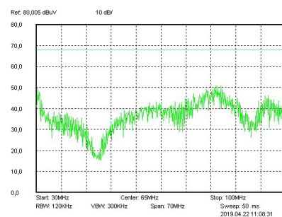
Рис. 67. Диапазон 30–100 МГц.
