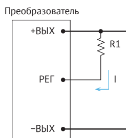
Рис. 4. Снижение U_{\text{вых.}}
