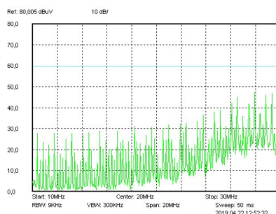
Рис. 69. Диапазон 10–30 МГц.
