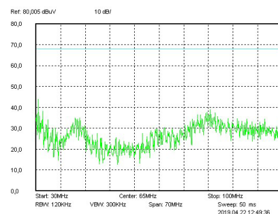
Рис. 70. Диапазон 30–100 МГц.
