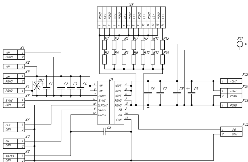
Рис. 3. Принципиальная электрическая схема демолат МНМ8-ДП-1И1,05,0; МНМ8-ДП-1В1,05,0.
