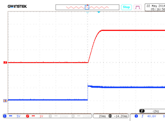
Рис. 12. Осциллограмма установления выходного напряжения с момента подачи входного напряжения. Луч 1 (синий) — входное напряжение. Масштаб 5 В/дел. Луч 2 (красный) — выходное напряжение. Масштаб 1 В/дел. Развертка 20 мс/дел.
