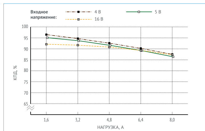
Рис. 30. КПД для МНМ8-1И1,05,0Т. (Выходное напряжение 3,3 В).
