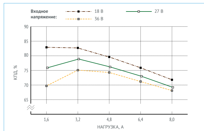
Рис. 19. КПД для МНМ8-1В1,05,0Т. (Выходное напряжение 1,2 В).
