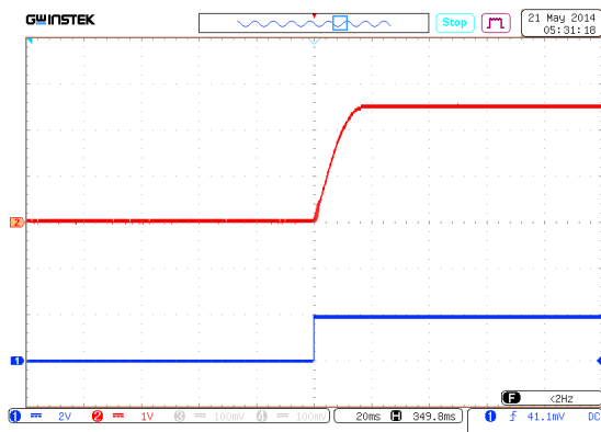
Рис. 6. Осциллограмма установления выходного напряжения с момента подачи команды дистанционного управления.
