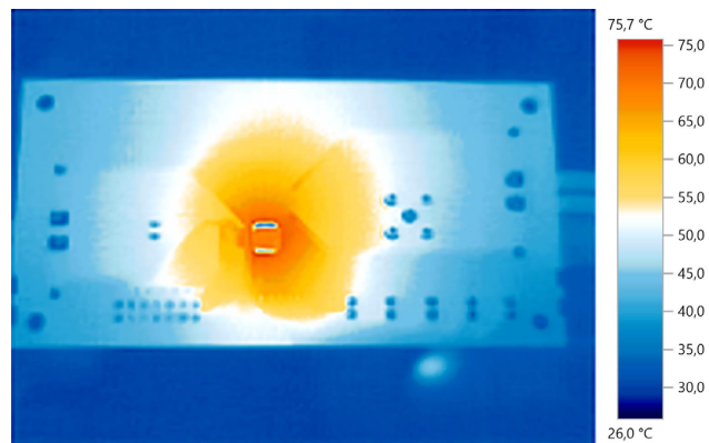
Рис. 38. Нижняя сторона. 69,4 °C
