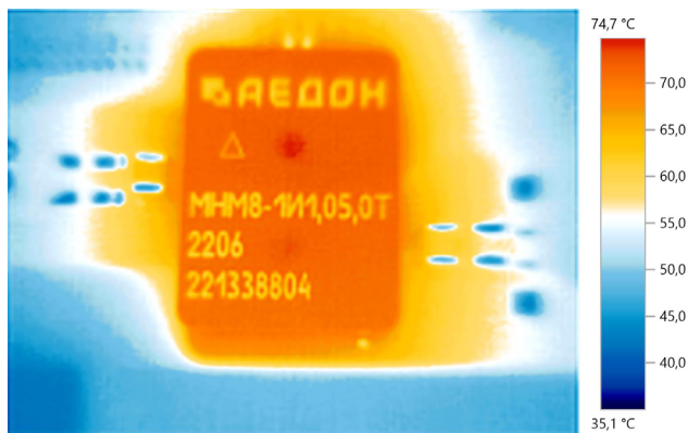
Рис. 37. Верхняя сторона. 74,7 °C
