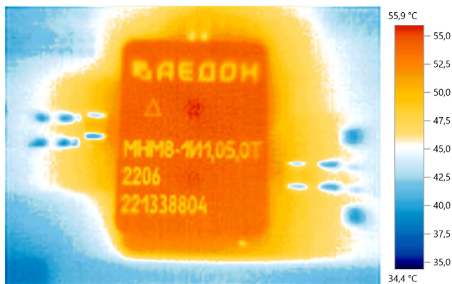
Рис. 35. Верхняя сторона. 55,9 °C
