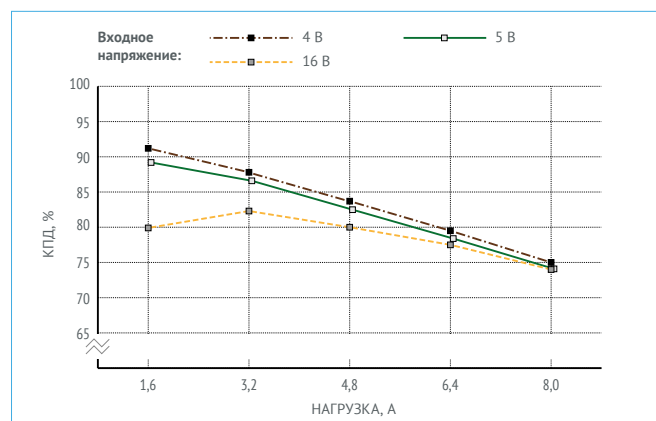
Рис. 26. КПД для МНМ8-1И1,05,0Т. (Выходное напряжение 1,2 В).
