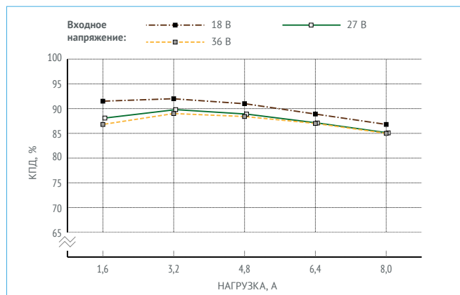
Рис. 23. КПД для МНМ8-1В1,05,0Т. (Выходное напряжение 3,3 В).
