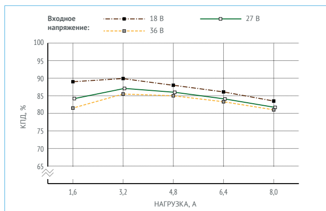
Рис. 21. КПД для МНМ8-1В1,05,0Т. (Выходное напряжение 2,5 В).
