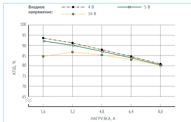
Рис. 28. КПД для МНМ8-1И1,05,0Т. (Выходное напряжение 1,8 В).
