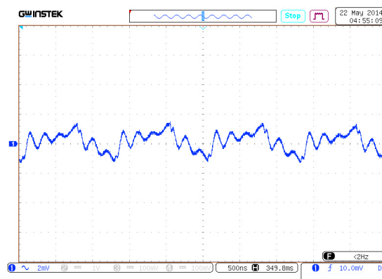
Рис. 14. Осциллограмма пульсаций выходного напряжения модуля при I_{OUT} = 8 А. Масштаб 2 мВ/дел. Развертка 500 нс/дел.
