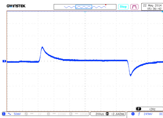
Рис. 13. Осциллограмма переходного отклонения выходного напряжения при изменении выходного тока. Масштаб 50 мВ/дел. Развертка 200 мкс/дел.
