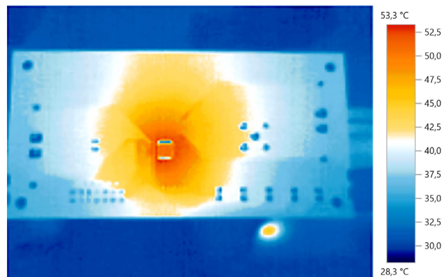
Рис. 36. Нижняя сторона. 50,7 °C
