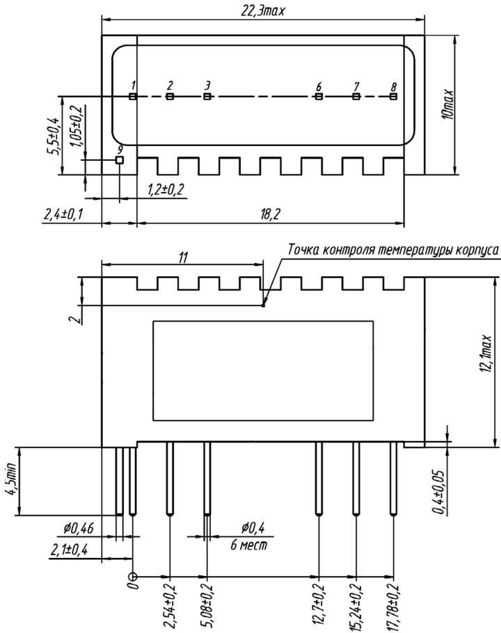
Рис. 32. Габаритный чертеж для МДМ10-Н.
