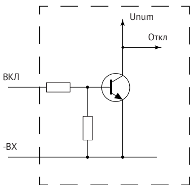
Рис. 3. Упрощенная схема цепи управления.
