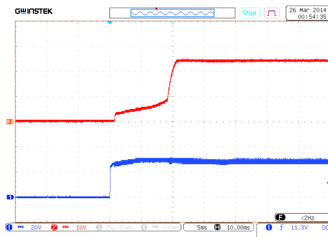
Рис. 18. Осциллограмма установления выходного напряжения с момента подачи входного напряжения.
