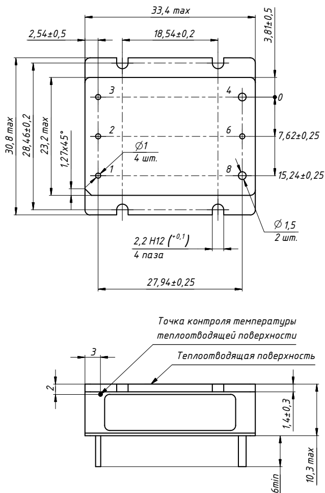
Рис. 21. Исполнение МДМ50-С.
