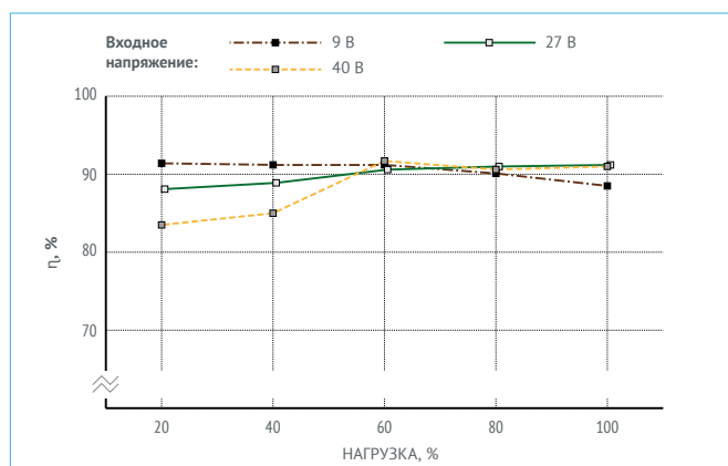
Рис. 10. МДМ50-1Б05РДС.
