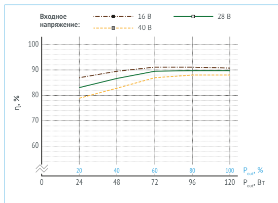
Рис. 15. МДМ120-1В27РДС.
