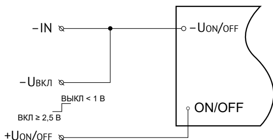
Рис. 7. Управление логическим напряжением.
