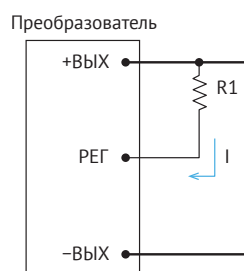
Рис. 9. Регулировка снижением U_{вых} .
