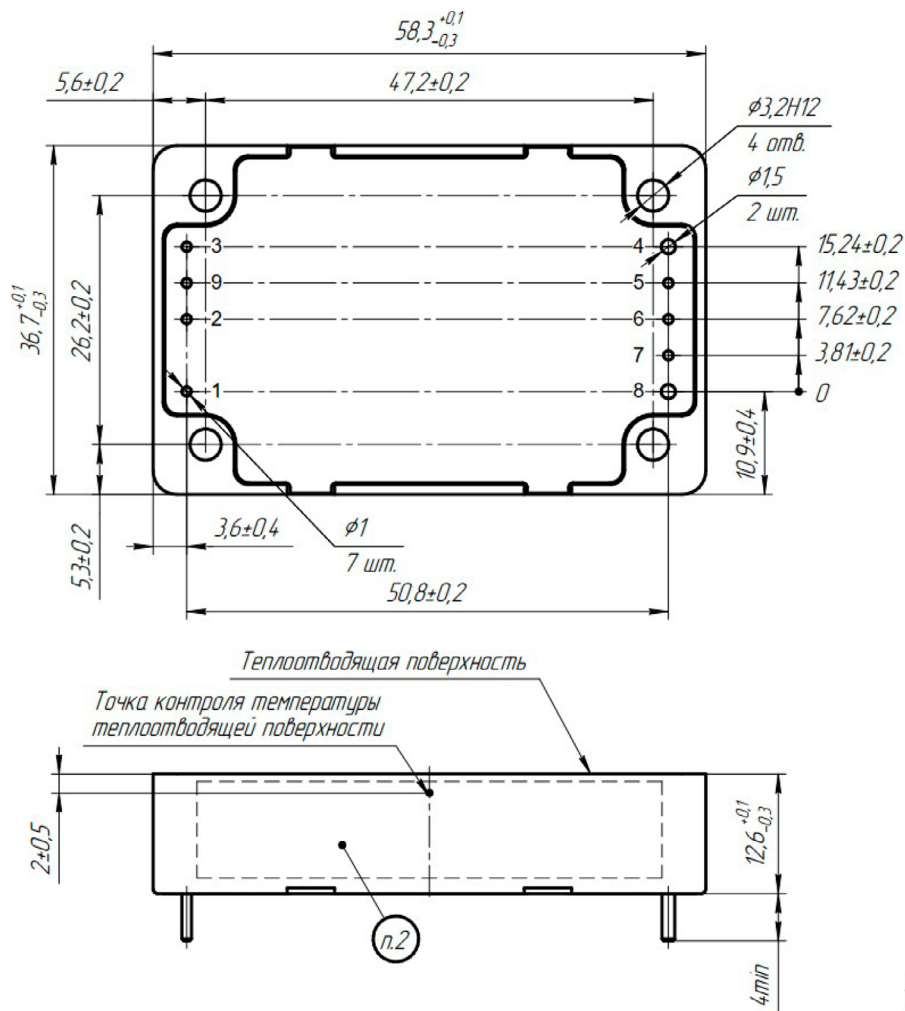
Рис. 22. Исполнение МДМ200-С.
