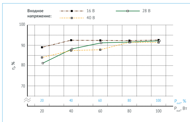
Рис. 14. МДМ200-1В12РС.
