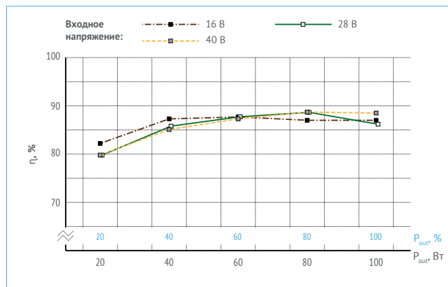
Рис. 16. МДМ200-1В24РС.
