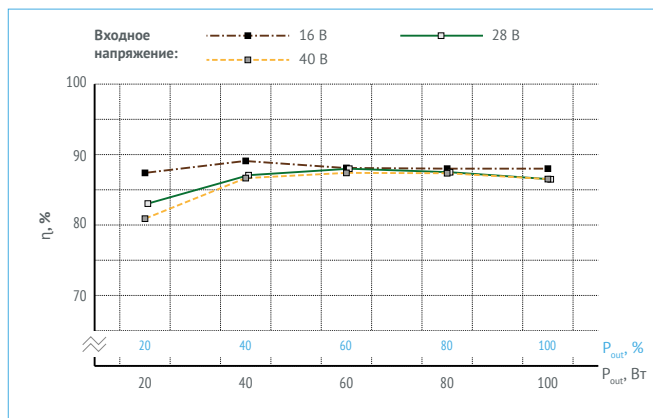
Рис. 15. МДМ200-1В15РС.
