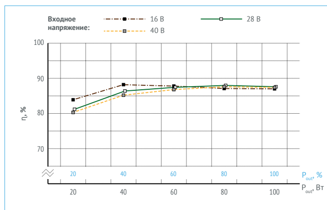
Рис. 17. МДМ200-1В27РС.
