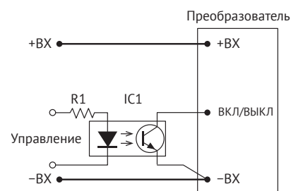
Рис. 6. ON/OFF с помощью оптрона.
