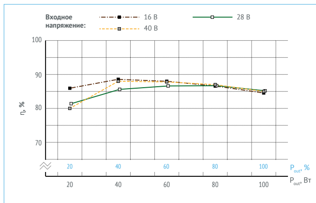
Рис. 13. МДМ200-1В05РС.
