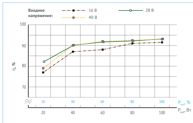
Рис. 18. МДМ200-1В48РС
