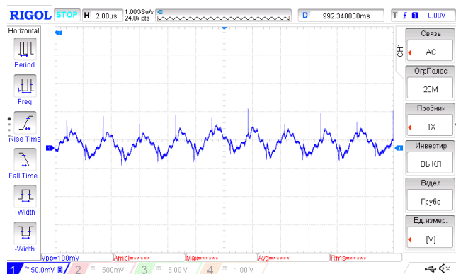
Рис. 21. Осциллограмма пульсаций U_{вых,ном} . Масштаб 50 мВ/дел. Развертка 2 мкс/дел.
