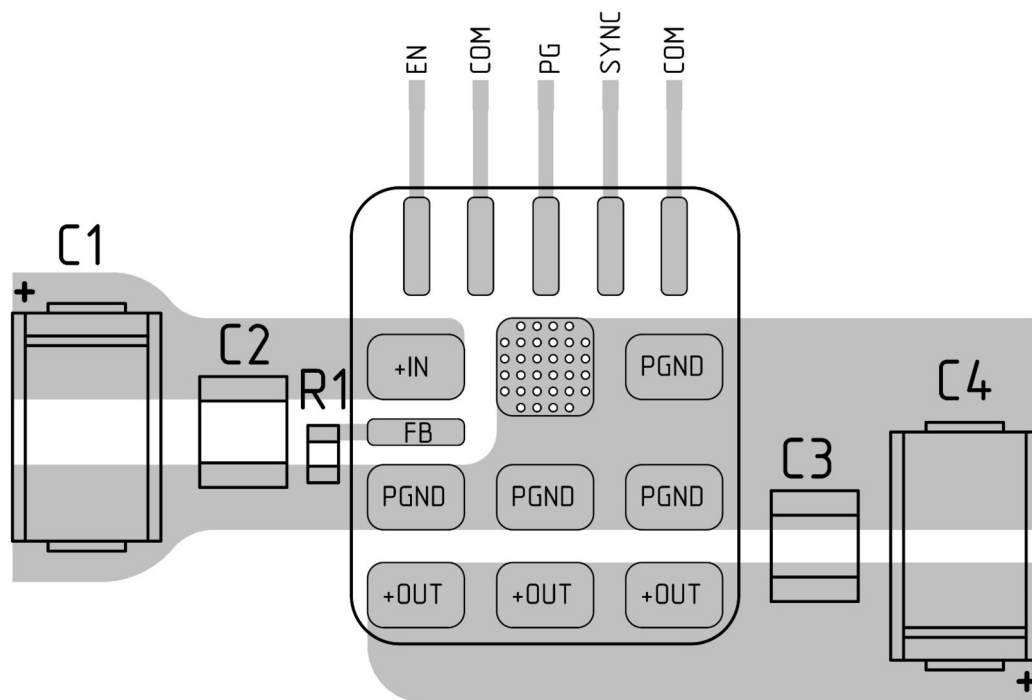
Рисунок Ж.1 — MNM1,2. Типовая топология
