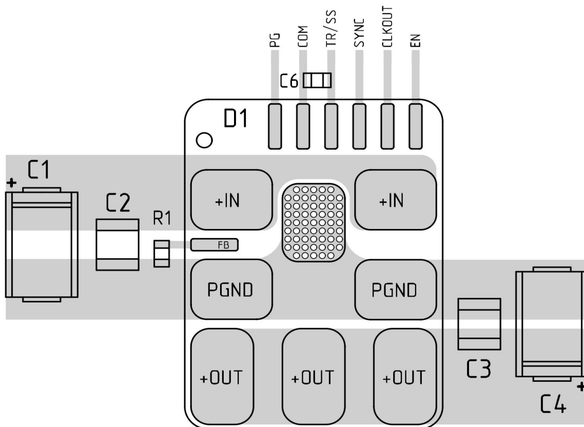
Рисунок Ж.3 — MHM8. Типовая топология
