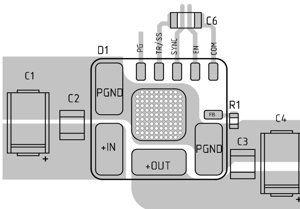
Рисунок Ж.2 — MNM4. Типовая топология
