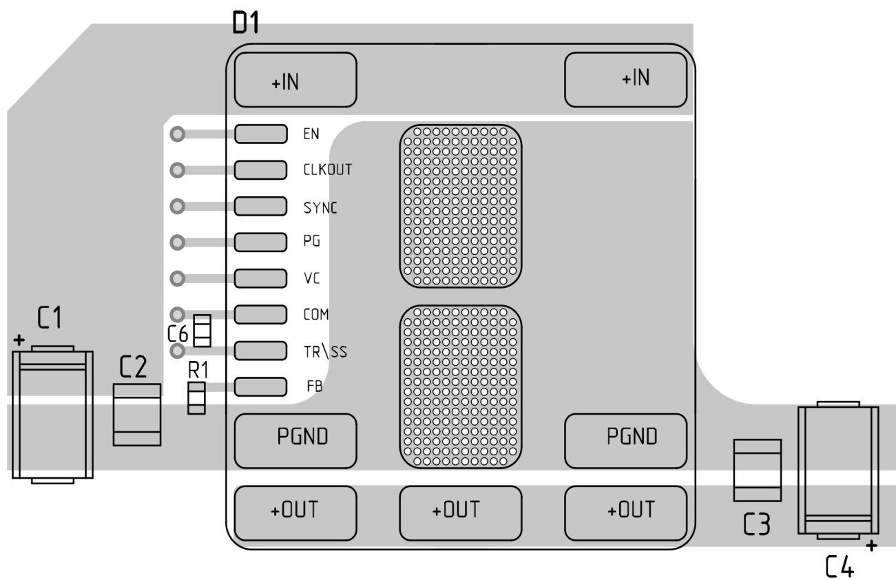
Рисунок Ж.4 — MHM15. Типовая топология
