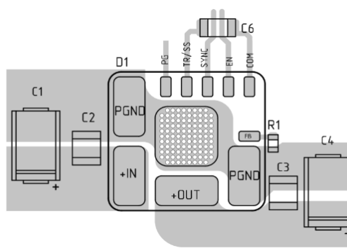
Рис. 4. Рекомендуемая топология печатной платы
