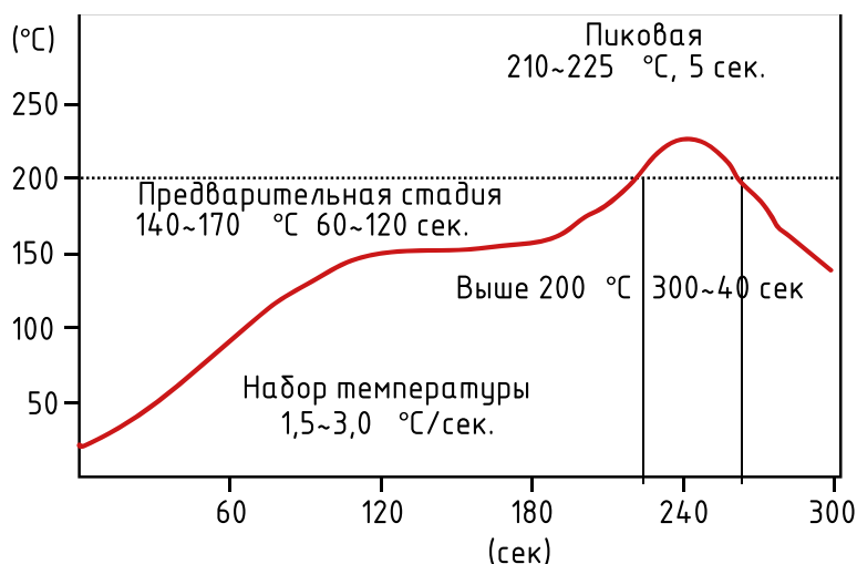
Рис. 5. Профиль оплавления
